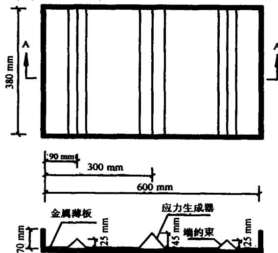
A-A 剖面 图 1 试验装置
