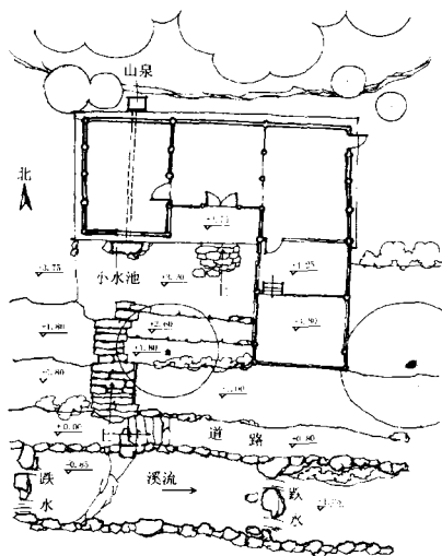
图3 吴宅平面图
